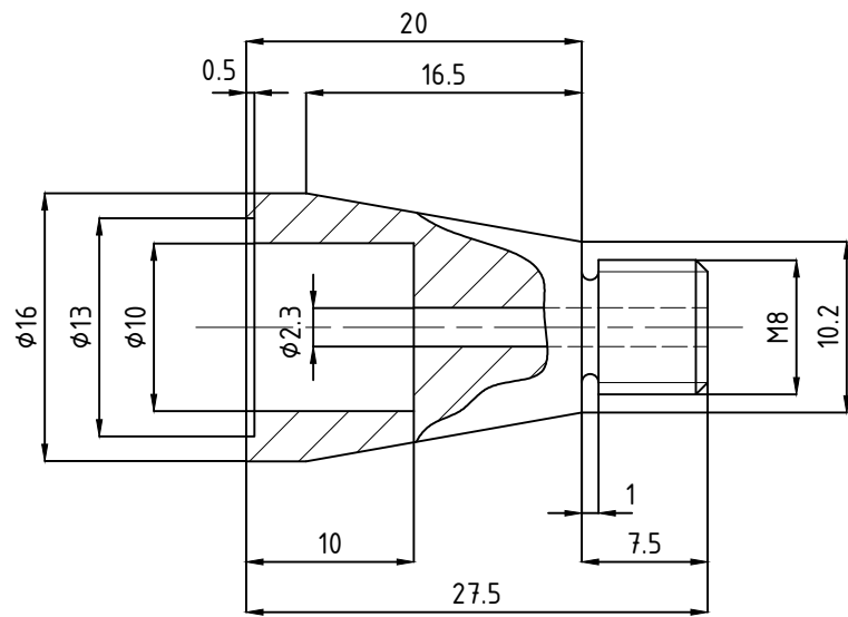
POS. 3 - AANSLUITSTUK BALLON
